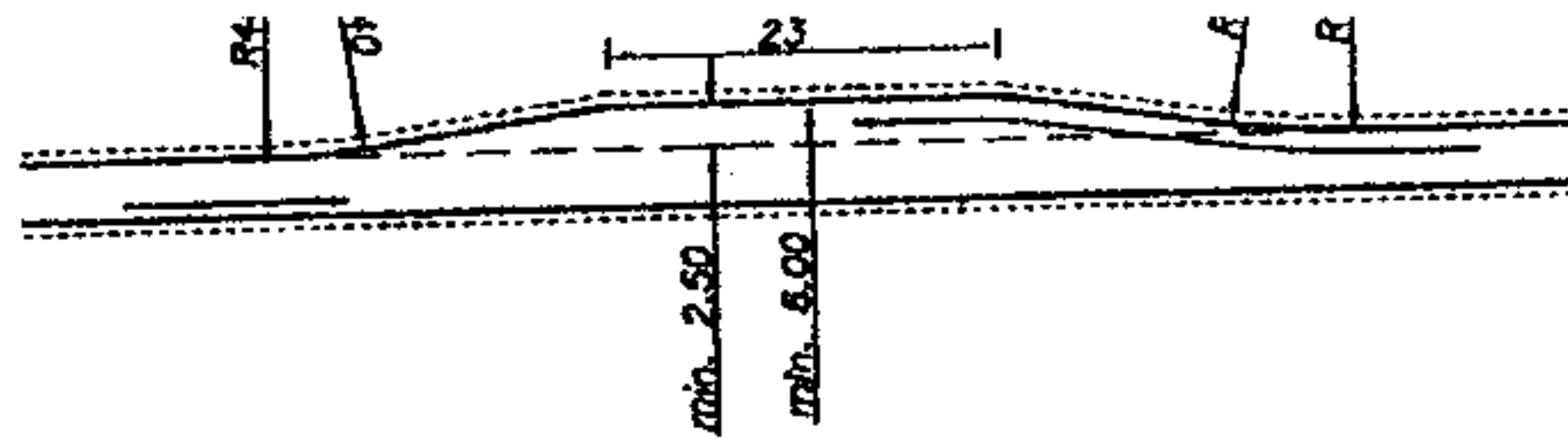
Rys.1. Mijanka drogowa na odcinku prostym
