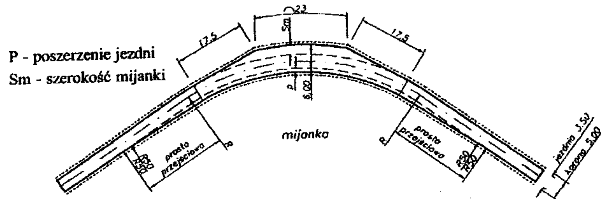
Rys.2. Mijanka drogowa na zewnętrznej stronie łuku
